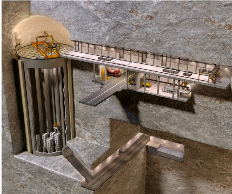
Figur 5-3. Siloförvaret i befintligt SFR under driftskedet.
