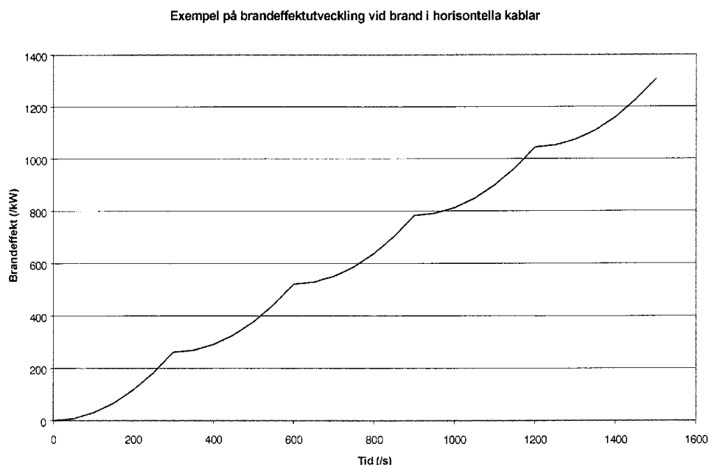
Figur 5 Effektutvecklingskurva vid brand i horisontell kabelstege. Vid endast en kabelstege blir effektutvecklingen konstant vid 220 kW osv.
