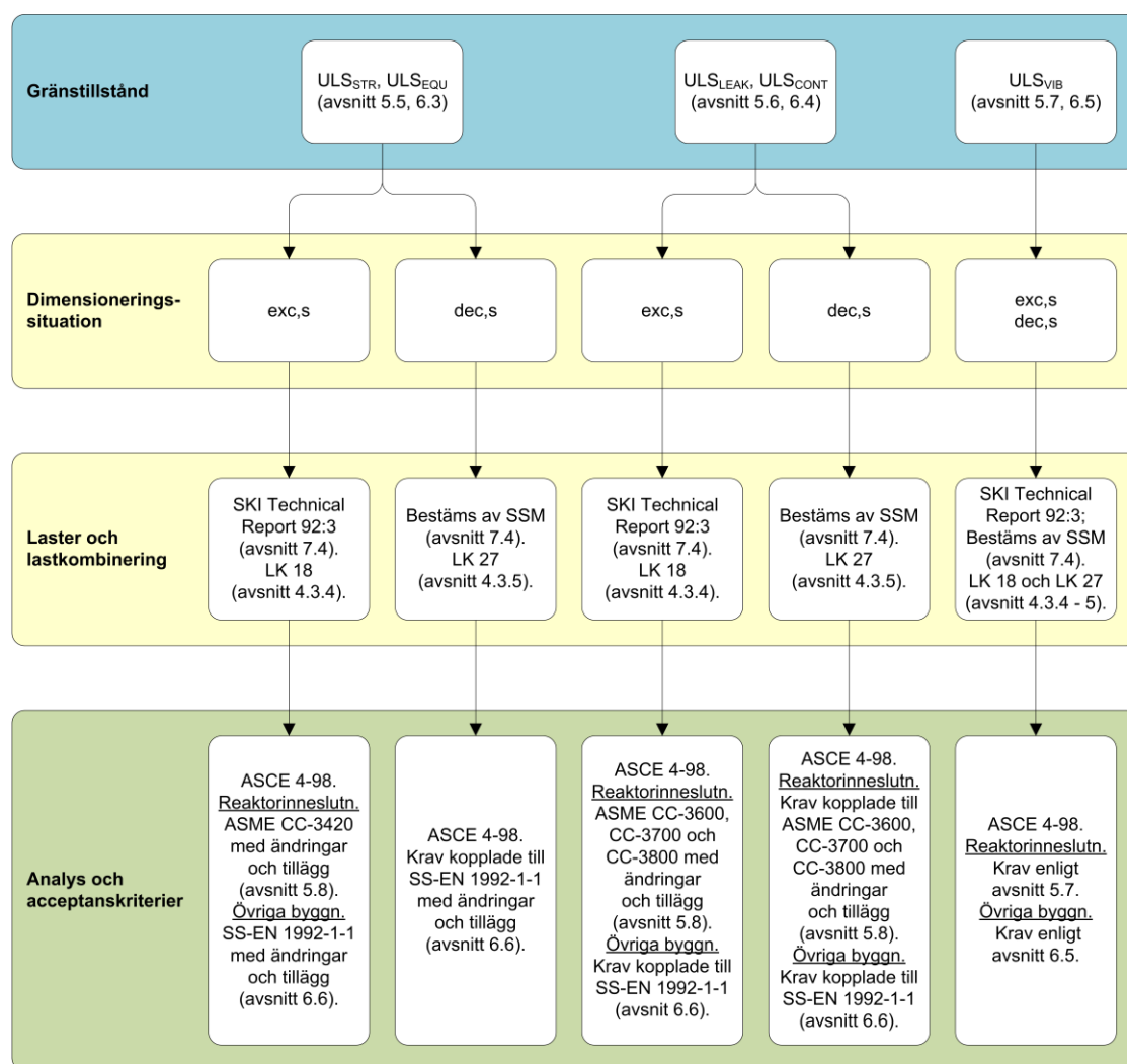
Figur 7.1 – Sammanfattning av dimensioneringsanvisningar med avseende på jordbävning.
